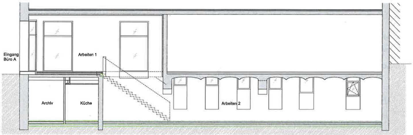
längsschnitt
